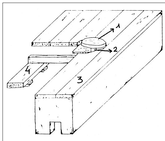
Torno de alfarero: 1. Rueda. 2. Árbol. 3. Tablero. 4. Taburete o banquillo
